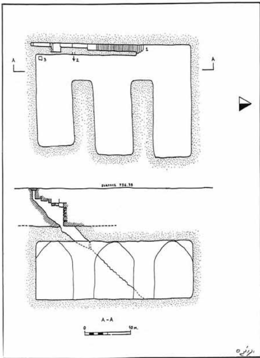
البئر رقم (5) مخطط البئر تم اعداده من قبل ورن عام 1867م رقم (1) درج (2) مدخل للبئر موجود في سقف البئر (3) مدخل للصهرج
